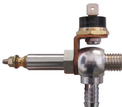
DH Schraub-/Filterversion
